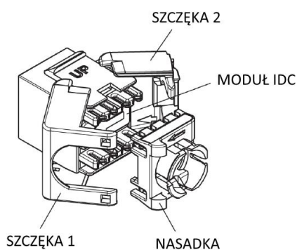
A. Widok z tyłu modułu Keystone
