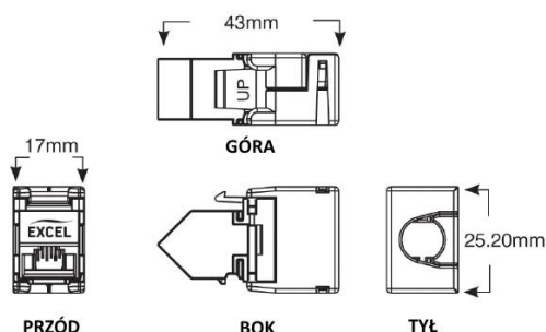
B. Profile modułu Keystone
