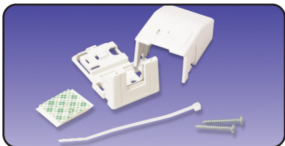
MX-SM1-(XX) ..... puszka 1-portowa z pokrywą, podstawą, jedną 1-portową osłoną MAX, opaskami kablowymi i wkrętami
